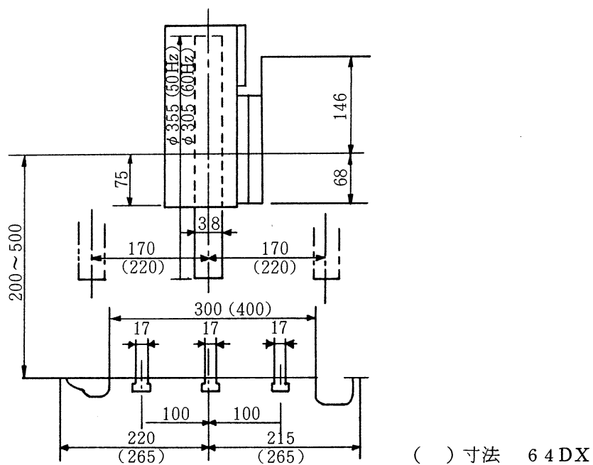
加工範囲図
