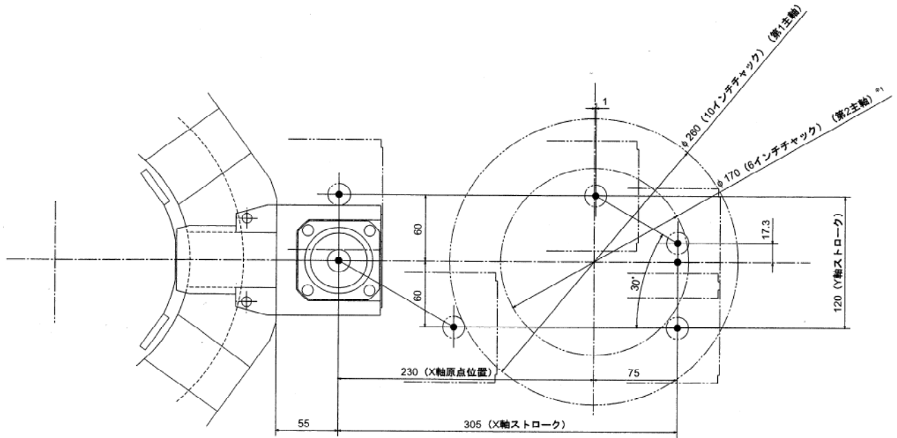
端面用回転工具刃先移動領域
