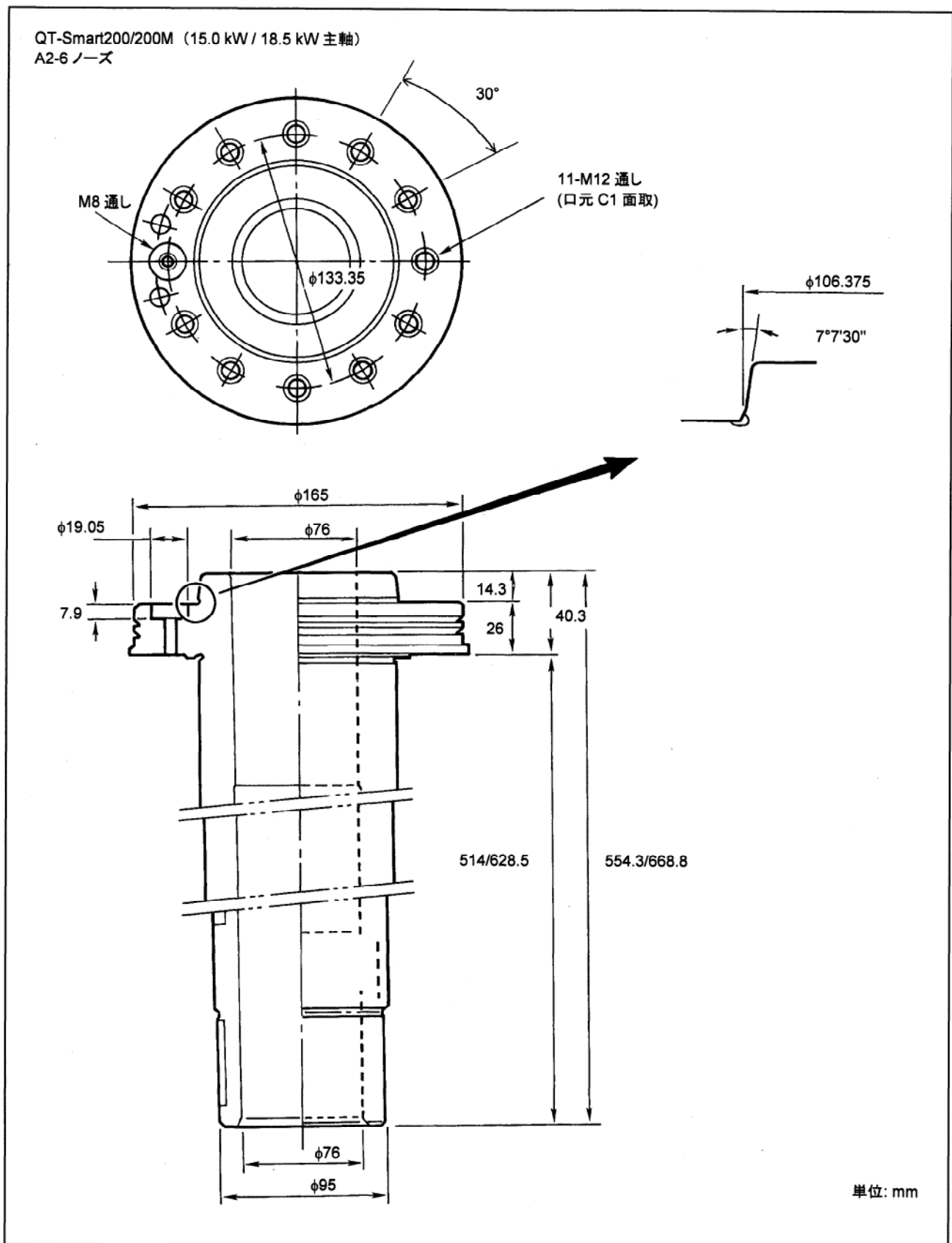
Fig. 9-1 主軸端図
