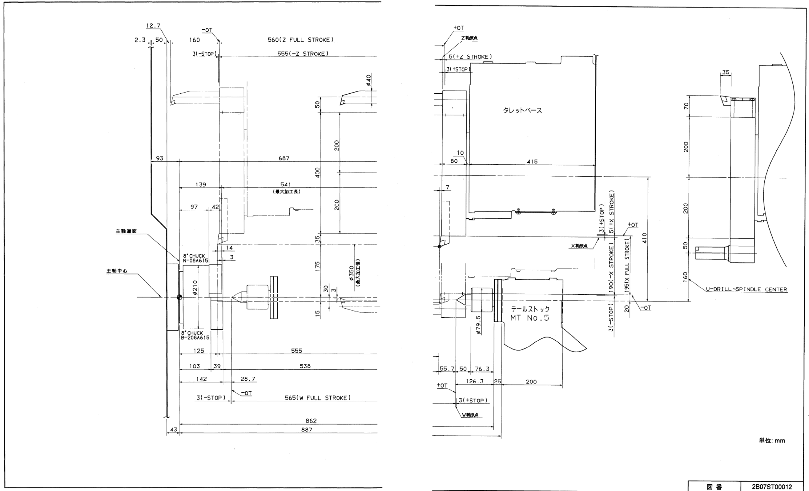
Fig. 9-5 ストローク線図 QT-Smart200
